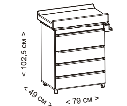
ВАННОЧКА MARTHA B-1971
