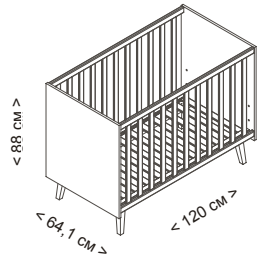
КРОВАТКА MARTHA 120x60
