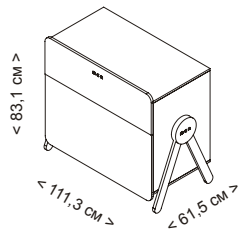
КОМОД SWING CO-1836
