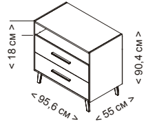
КОМОД TREVI CO-1959
